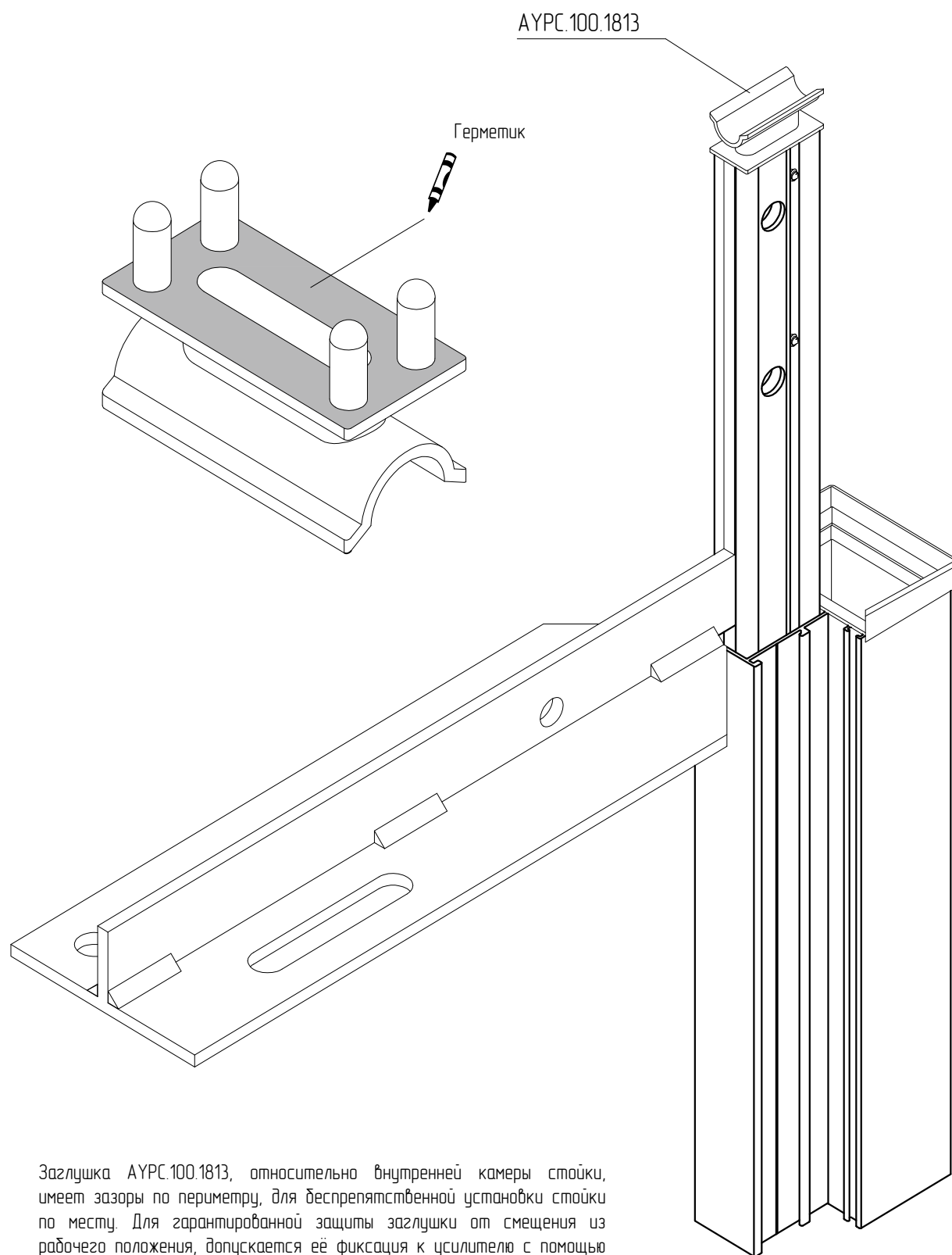
Схема установки заглушек влагоотвода АУРС.100.1813 и АУРС.100.1814
