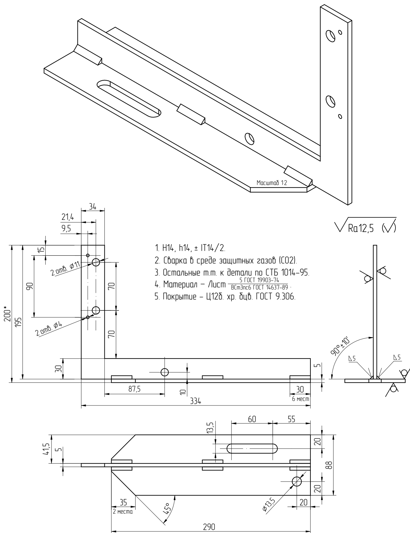
Кронштейн АУРС.100.1750 с размерами
