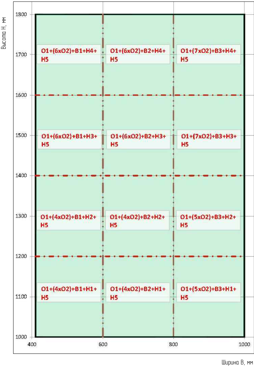
График для выбора размеров створки 100P.1303 из профилей АУРС.100Р (паз ПВХ) и поворотно-откидного комплекта фурнитуры ROTO (до 100 кг)
