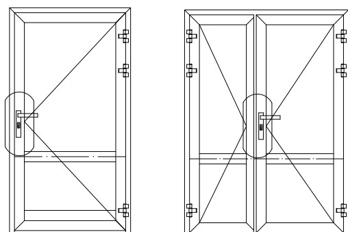
Схема установки ответной планки АУРС.W72.0975 под замок Stublina 3149.30/Р
