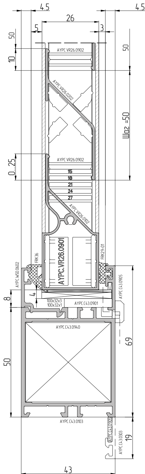
Окно-дверная система без терморазрыва ALT C43
