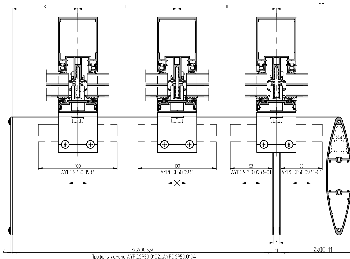
Доработка торцевой крышки AYPC.SP50.0802...AYPC.SP50.0804 под установку элемента сухарного AYPC.SP50.0933-01
