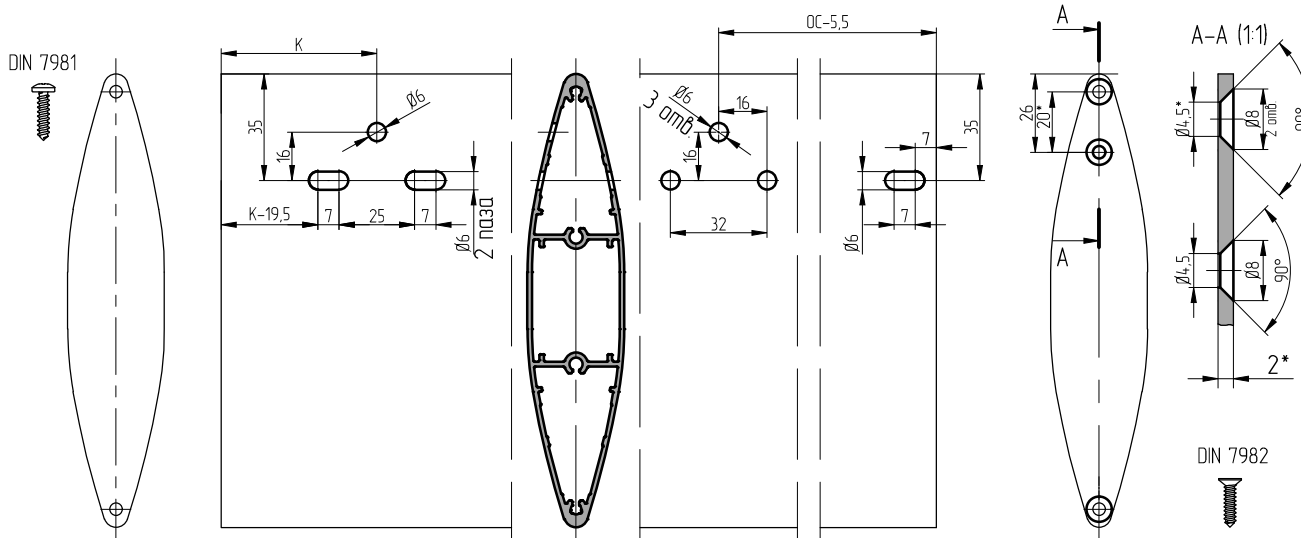
Торцевая крышка AYPC.SP50.0802...AYPC.SP50.0804
