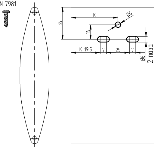
Торцевая крышка AYPC.SP50.0802...AYPC.SP50.0804
