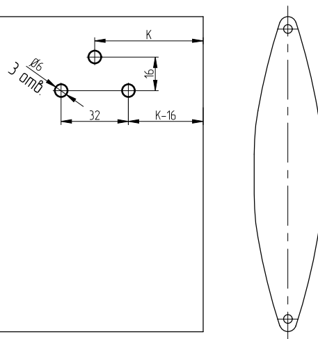
Торцевая крышка AYPC.SP50.0802...AYPC.SP50.0804
