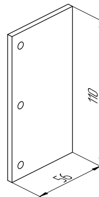
Пластина
