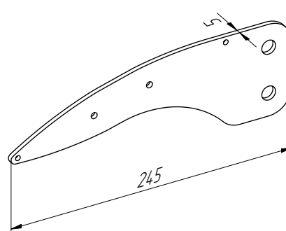
Торцевая крышка-кронштейн 15° для ламели 200 мм
