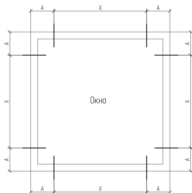
Схема расположения крепежных элементов
