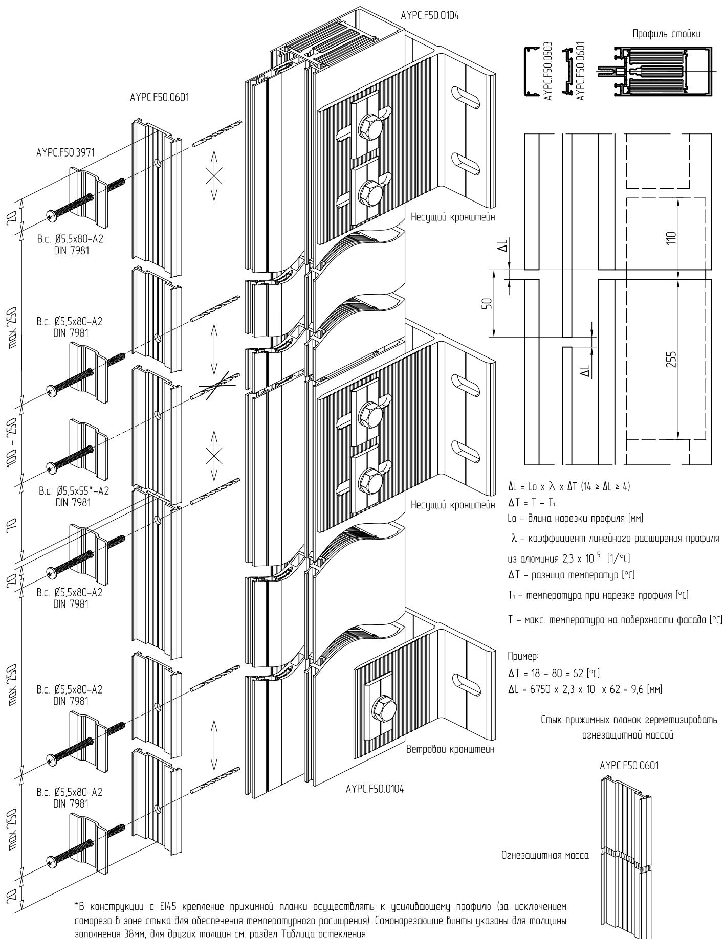
Схема расположения крепежных элементов на стойке EI 45.
