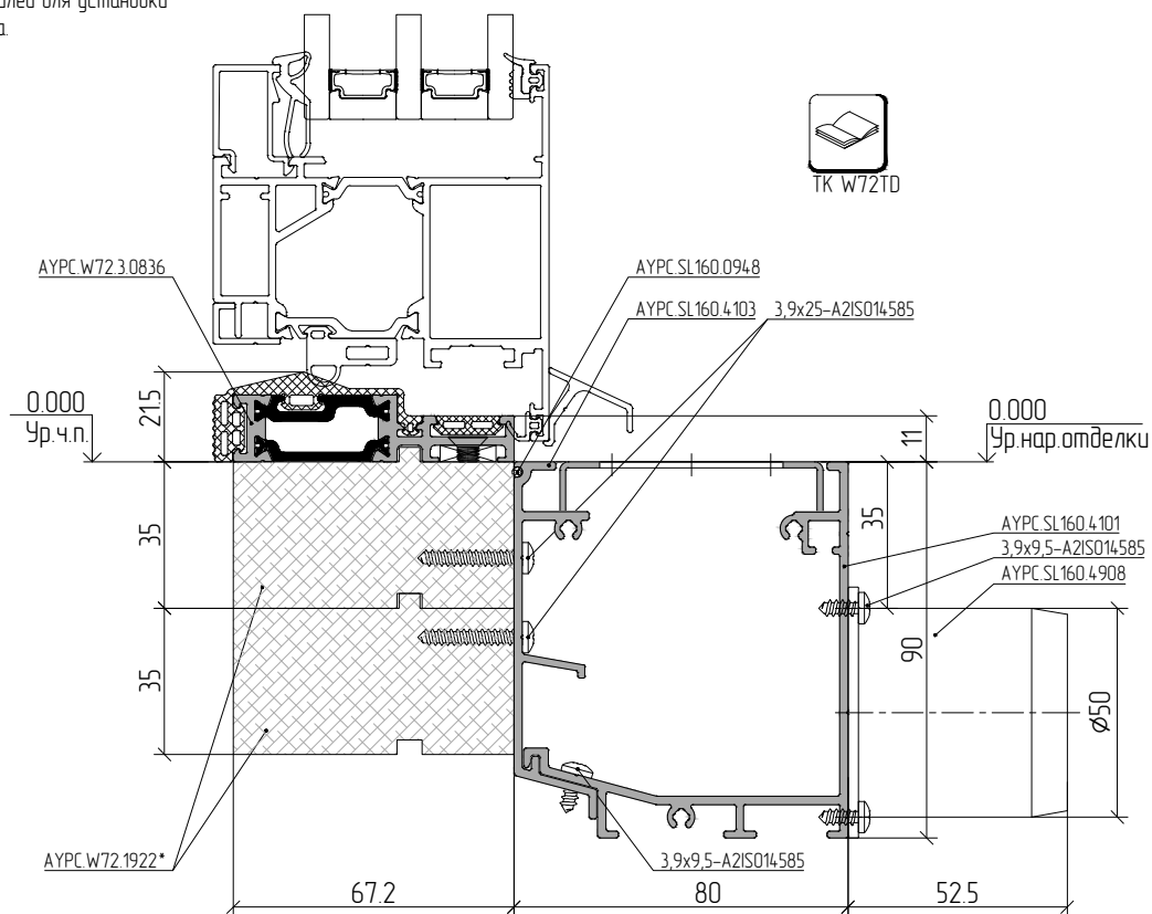
10a-10a
