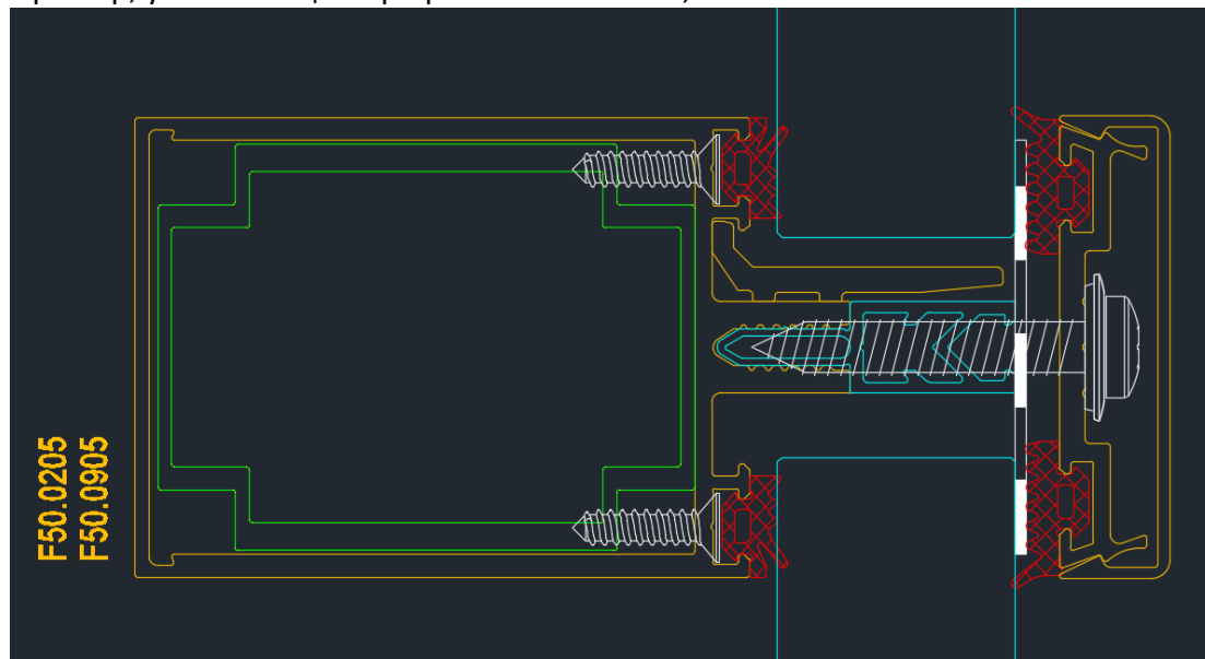
Пример, усиливающий профиль F50.0318 + 3,9x16-7982
