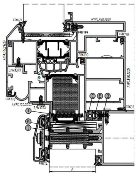
Сечение через ригель
