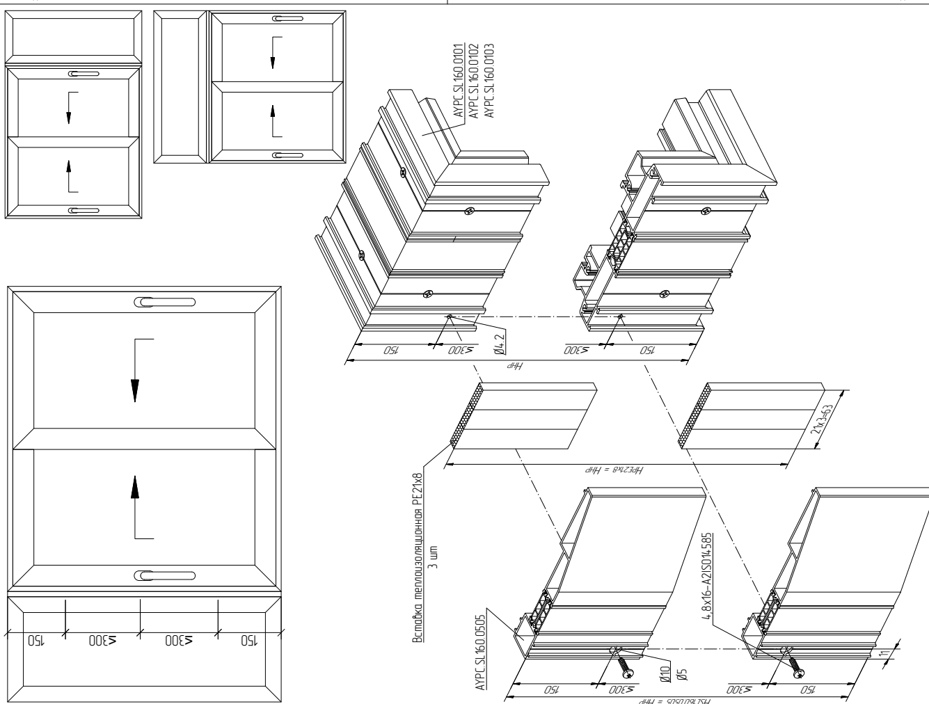
Интеграция подъемно-раздвижной конструкции с W62/W72. Шаг 1
