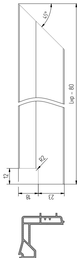
Обработка профиля водоотвода АУРС.СЛ160.0922
