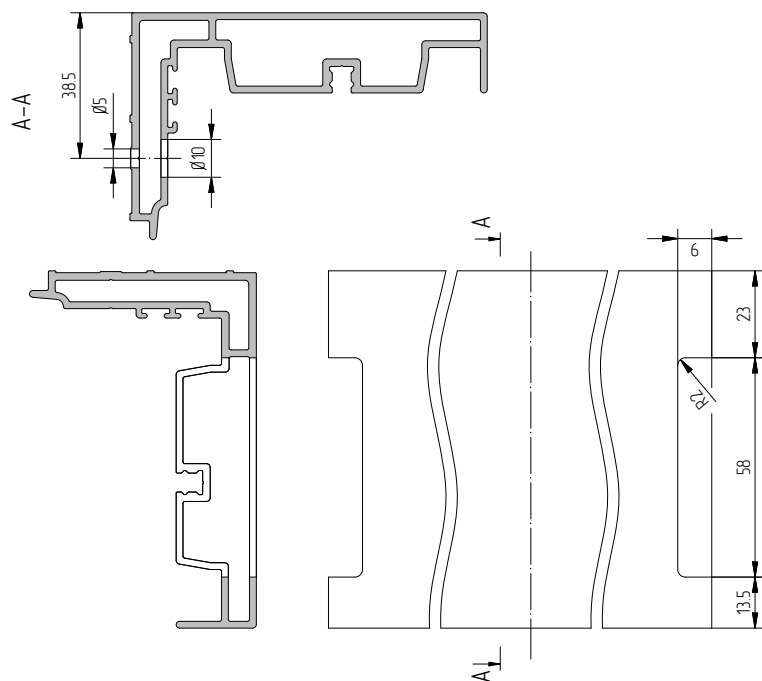
Схема обработки профиля прибора АУРС.SI.160.0813
