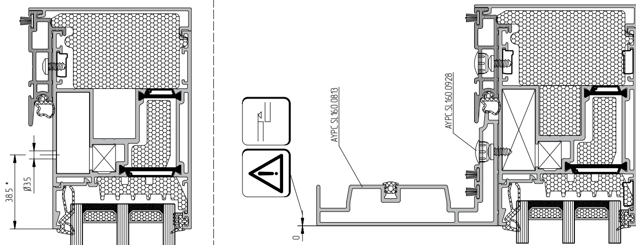
Схема обработки профиля створки
