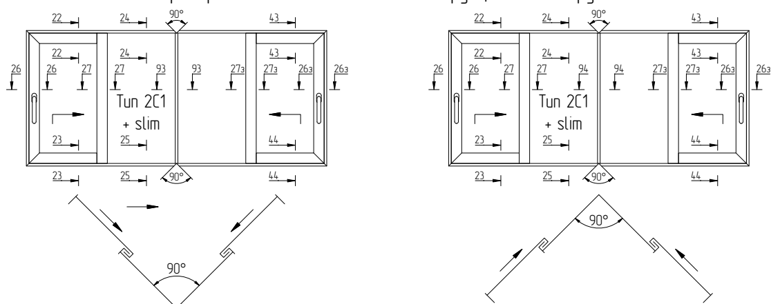
Примеры исполнения типовых конструкций. Вид снаружи
