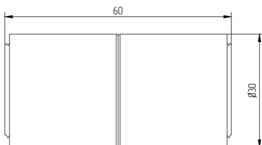
ДВРС-02 Магнитный улавливатель 60 мм
