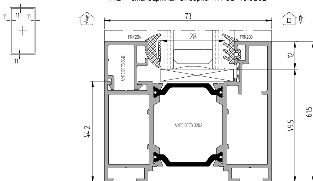
Сечение 11 – Створка А.2 – Стандартная створка АУРС.BF73.0202
