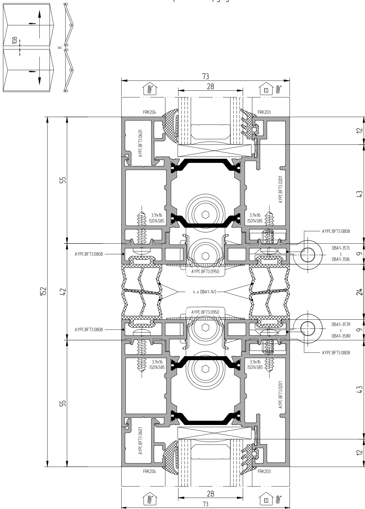
Сечение 10 – Фурнитурный узел К В.1 – Стык створок с адаптерами АУРС.BF73.0808 и полупетлями. Узкая створка АУРС.BF73.0201
