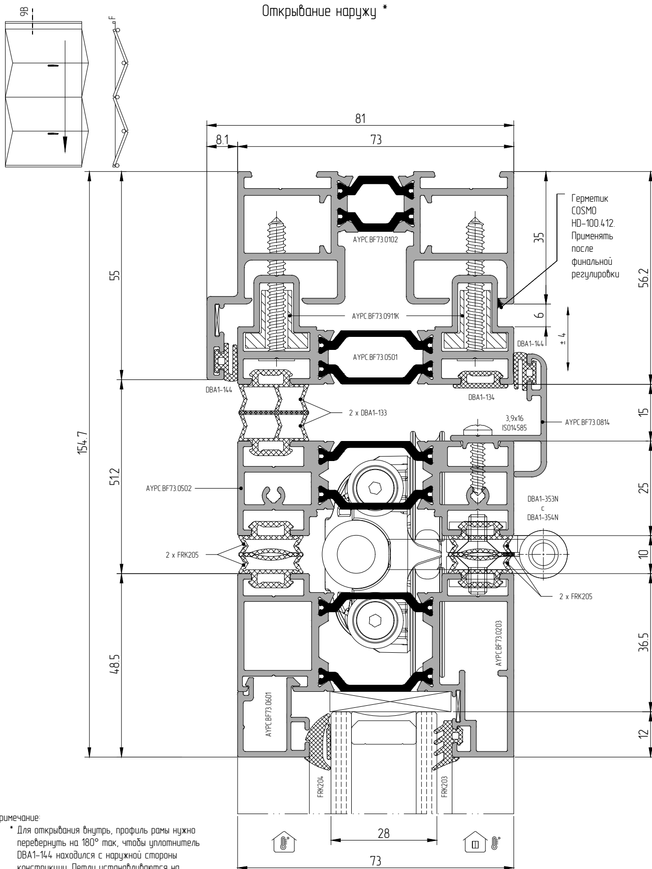
Сечение 9 – Фурнитурный узел F В.3 — Стык штульпа АУРС.BF73.0502 и регулирующего профиля. Сверхзская створка АУРС.BF73.0203
