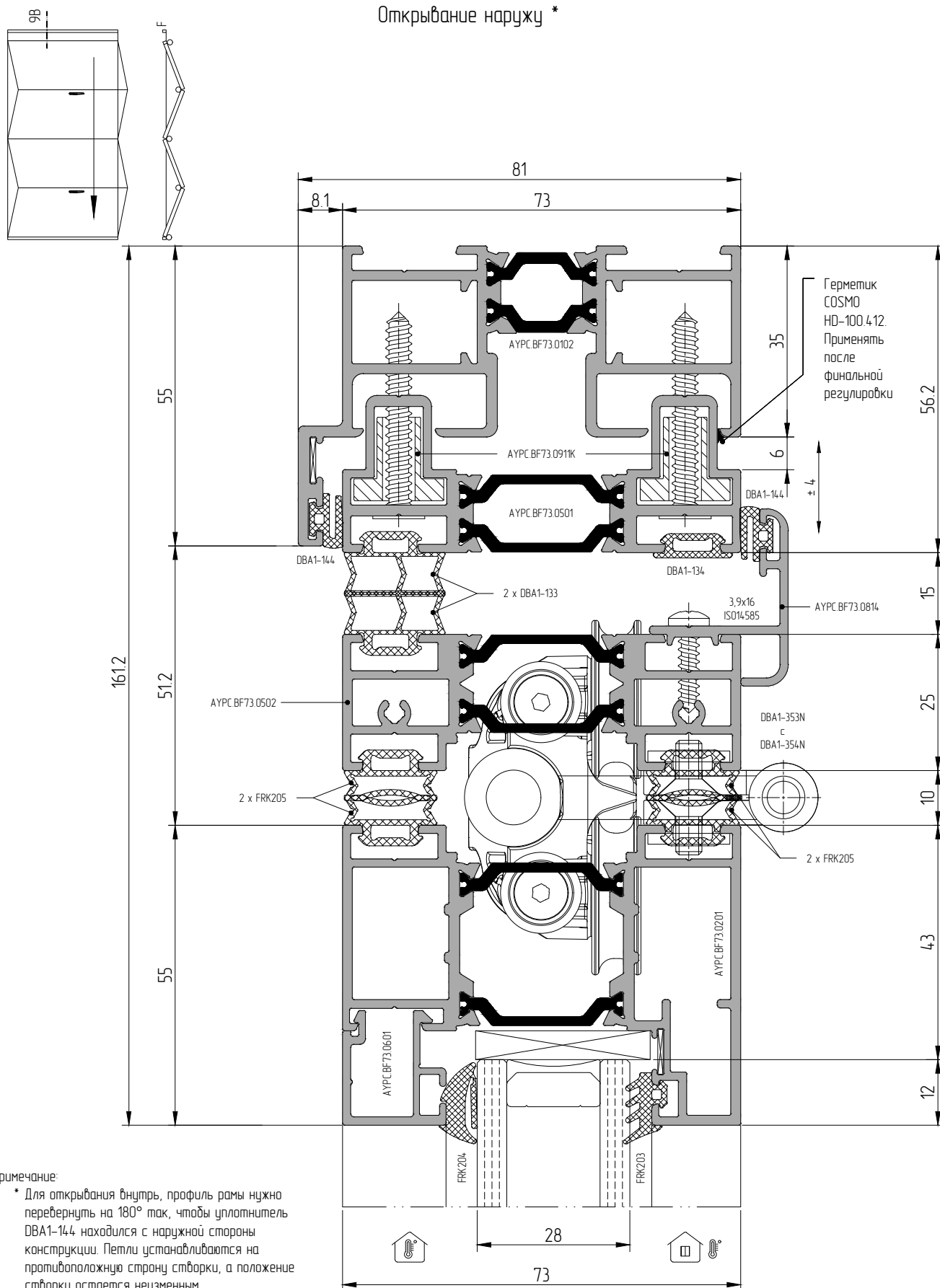
Сечение 9 – Фурнитурный узел F В.1 — Стык штульпа АУРС.BF73.0502 и регулировочного профиля. Узкая створка АУРС.BF73.0201
