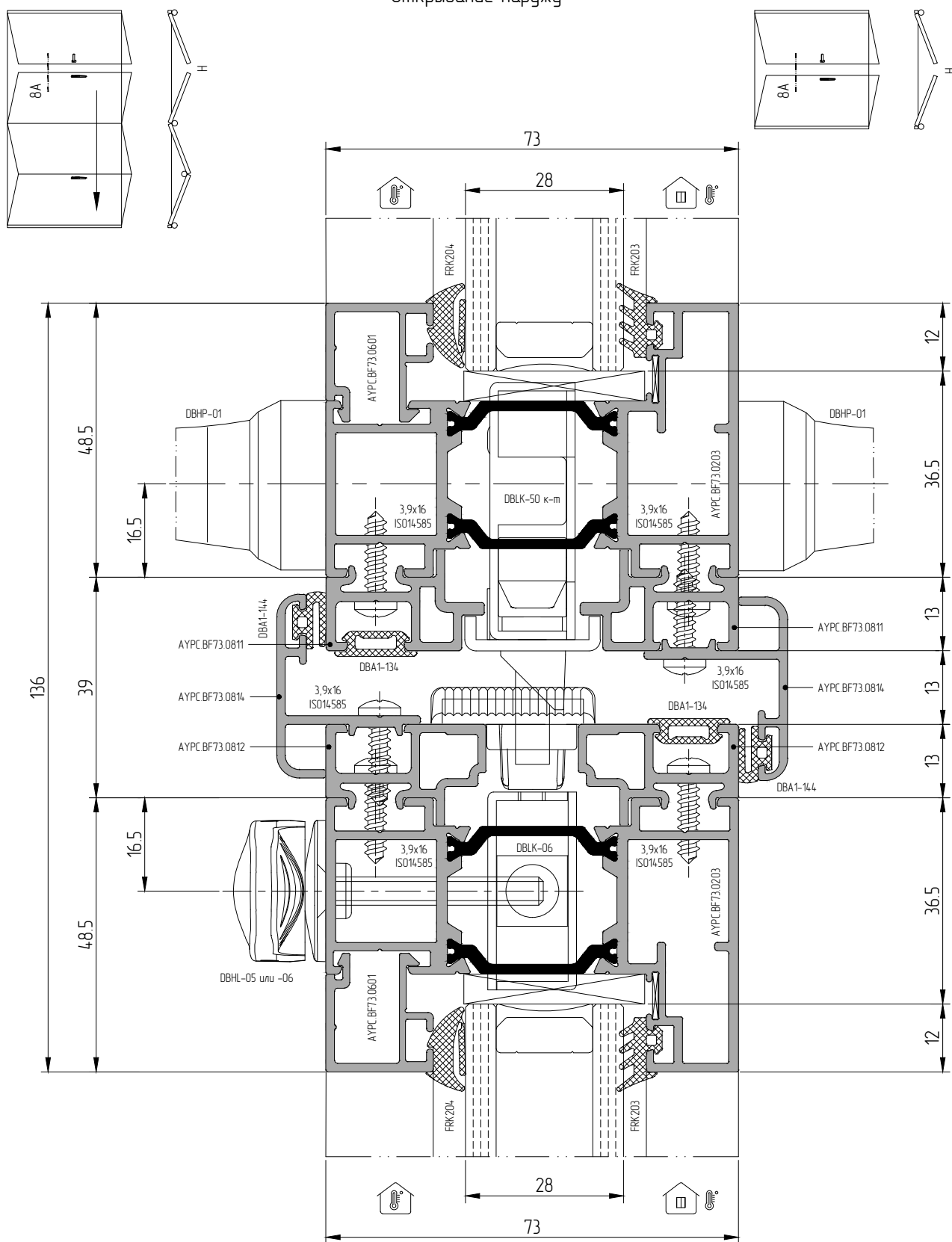
Сечение 8 – Фурнитурный узел Н А.3 – Стык створок с замком и шпингалетом. Сверхзужая створка АУРС.BF73.0203
