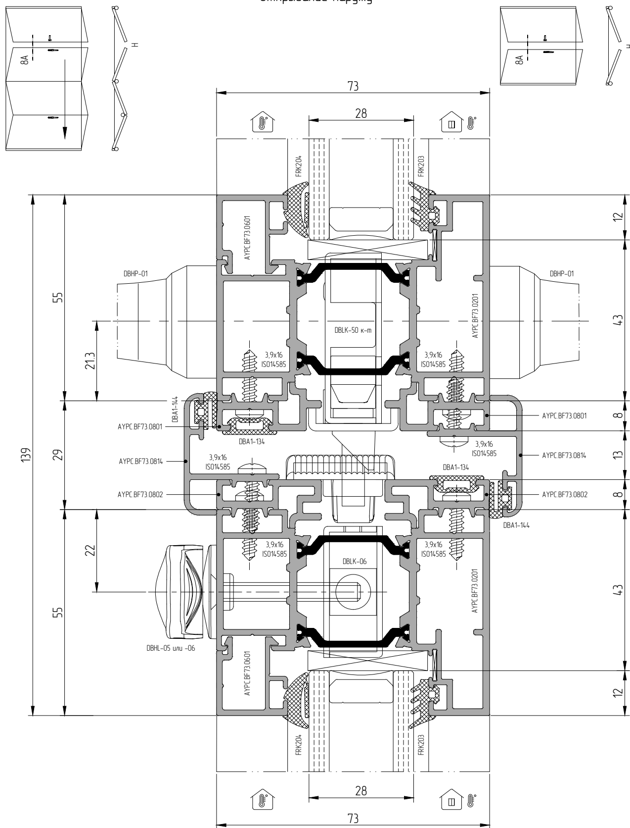
Сечение 8 – Фурнитурный узел Н А.1 — Стык створок с замком и шпингалетом. Узкая створка АУРС.BF73.0201
