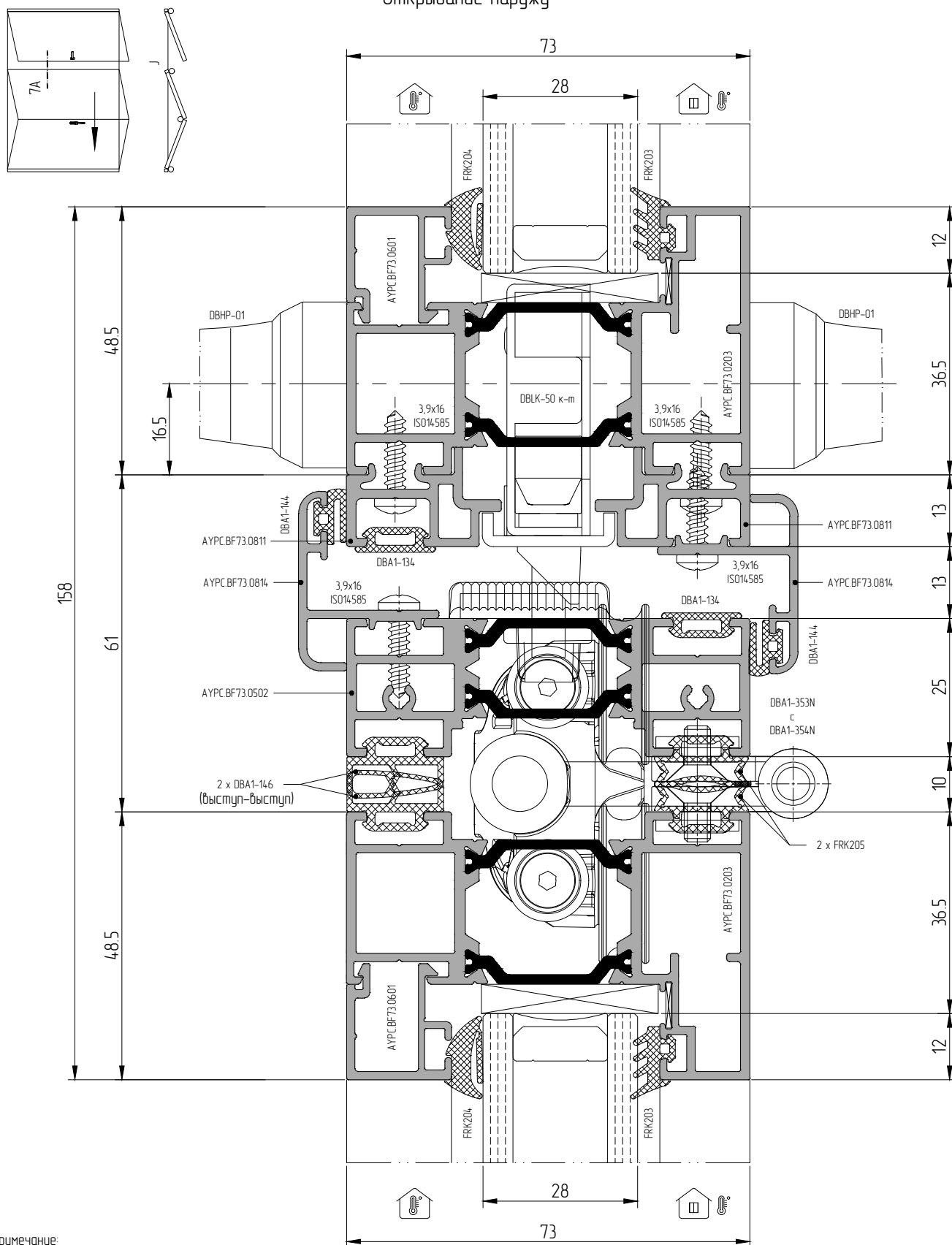
Сечение 7 – Фурнитурный узел J А.3 — Штульп АУРС.ВF73.0502 с ответной планкой замка. Сверхзская створка АУРС.ВF73.0203
