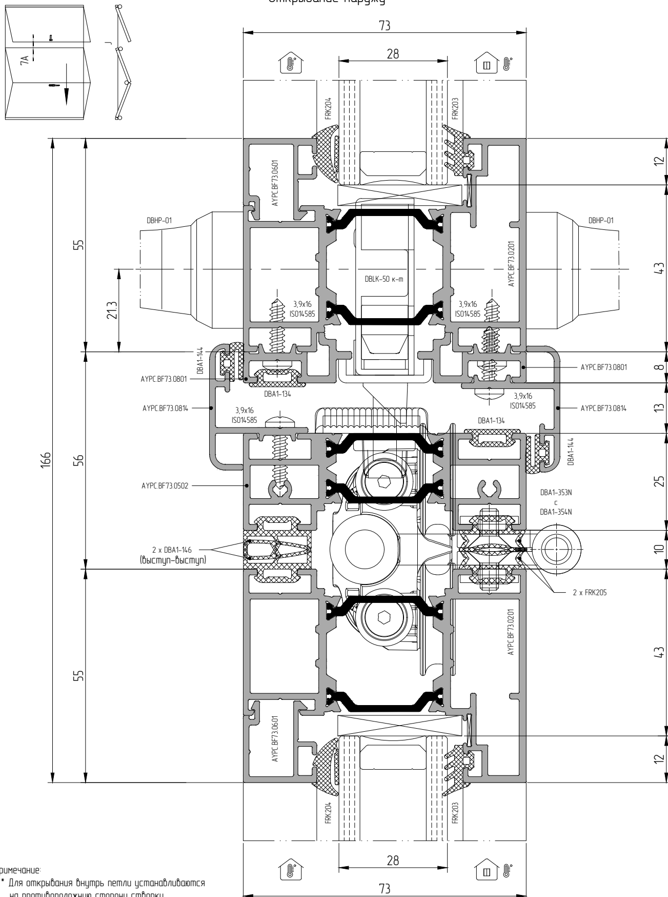
Сечение 7 – Фурнитурный узел J А.1 — Штульп АУРС.BF73.0502 с ответной планкой замка. Узкая створка АУРС.BF73.0201
