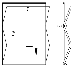
Сечение 5 – Фурнитурный узел Е А.3 — Стык створок с опорным и направляющим роликами. Сверхузкая створка АУРС.BF73.0203 Открывание наружу *
