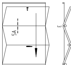
Сечение 5 – Фурнитурный узел Е А.1 — Стык створок с опорным и направляющим роликами. Узкая створка АУРС.BF73.0201 Открывание наружу *
