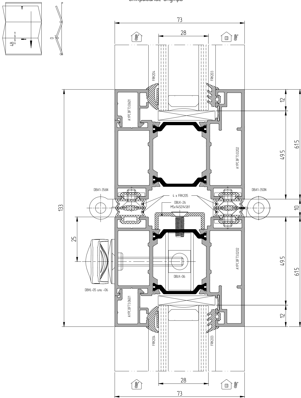
Сечение 4 – Фурнитурный узел D В.2 – Стык створок с петлей и шпингалетом. Стандартная створка АУРС.BF73.0202
