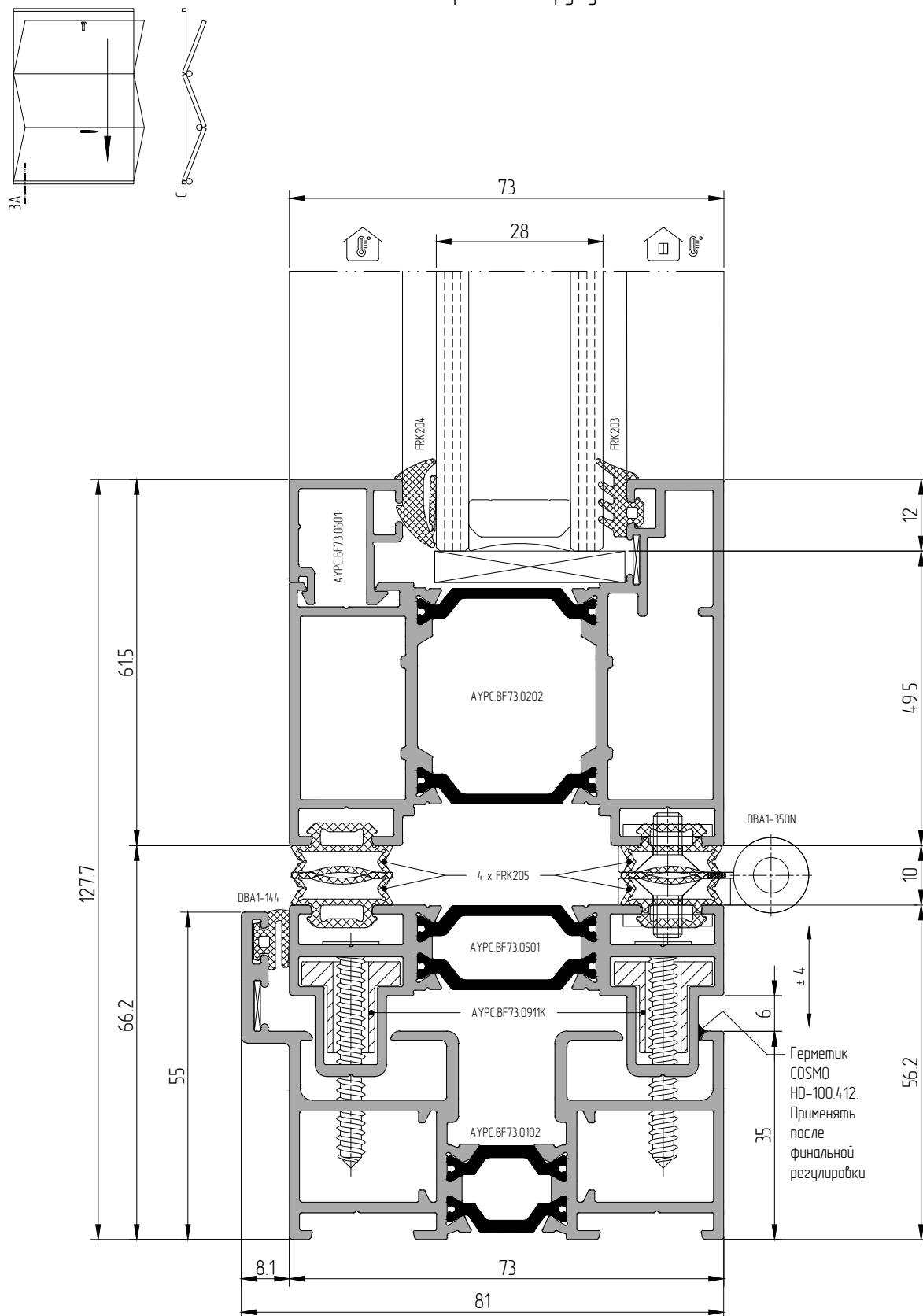
Сечение 3 – Фурнитурный узел С А.2 — Петли на регулирующем профиле АУРС.ВF73.0501. Стандартная створка АУРС.ВF73.0202
