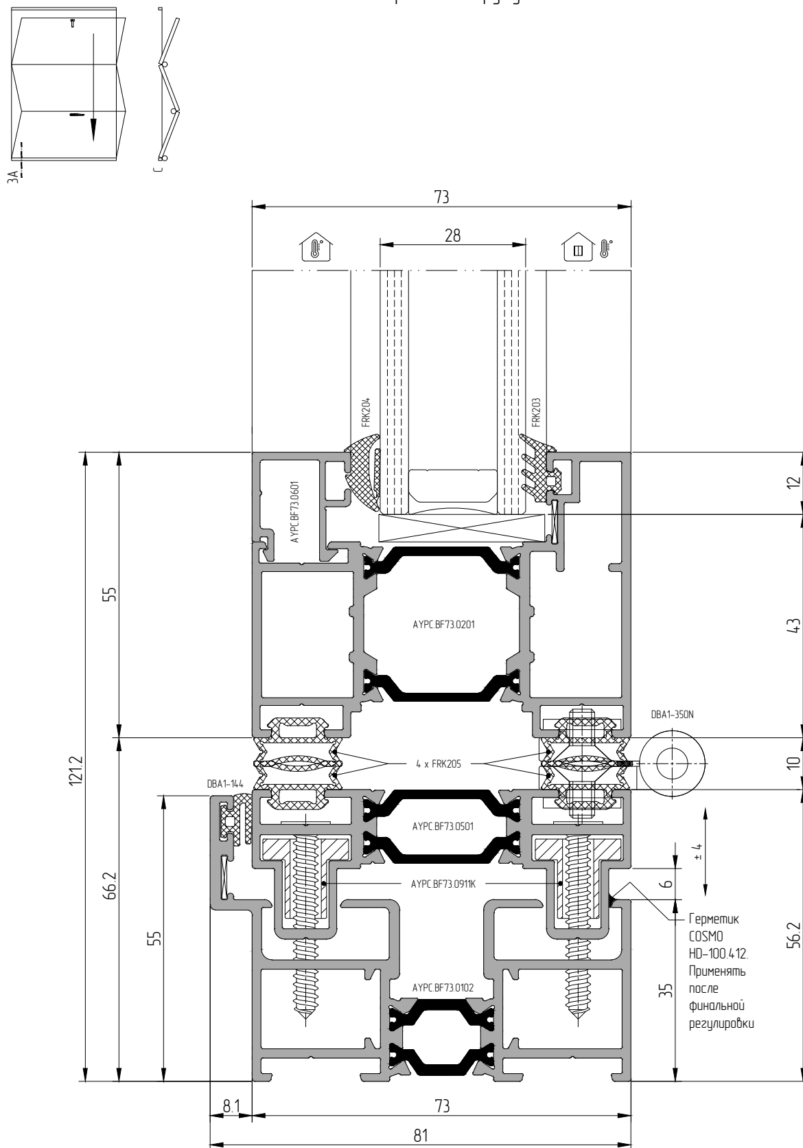
Сечение 3 – Фурнитурный узел С А.1 — Петли на регулирующем профиле АУРС.ВF73.0501. Узкая створка АУРС.ВF73.0201
