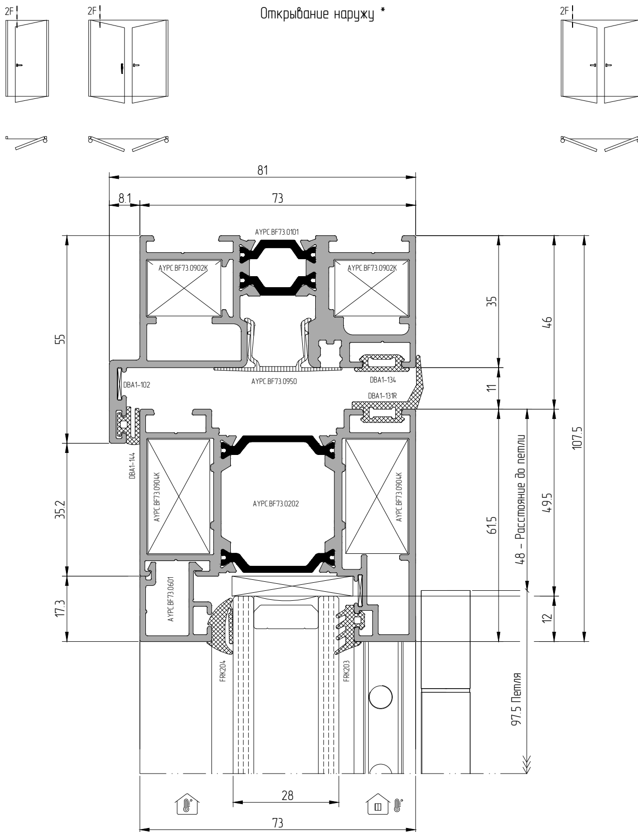
Сечение 2 – Верхний узел F.2 — Одностворчатые и двустворчатые двери. Верхний узел. Стандартная створка АУРС.ВФ73.0202
