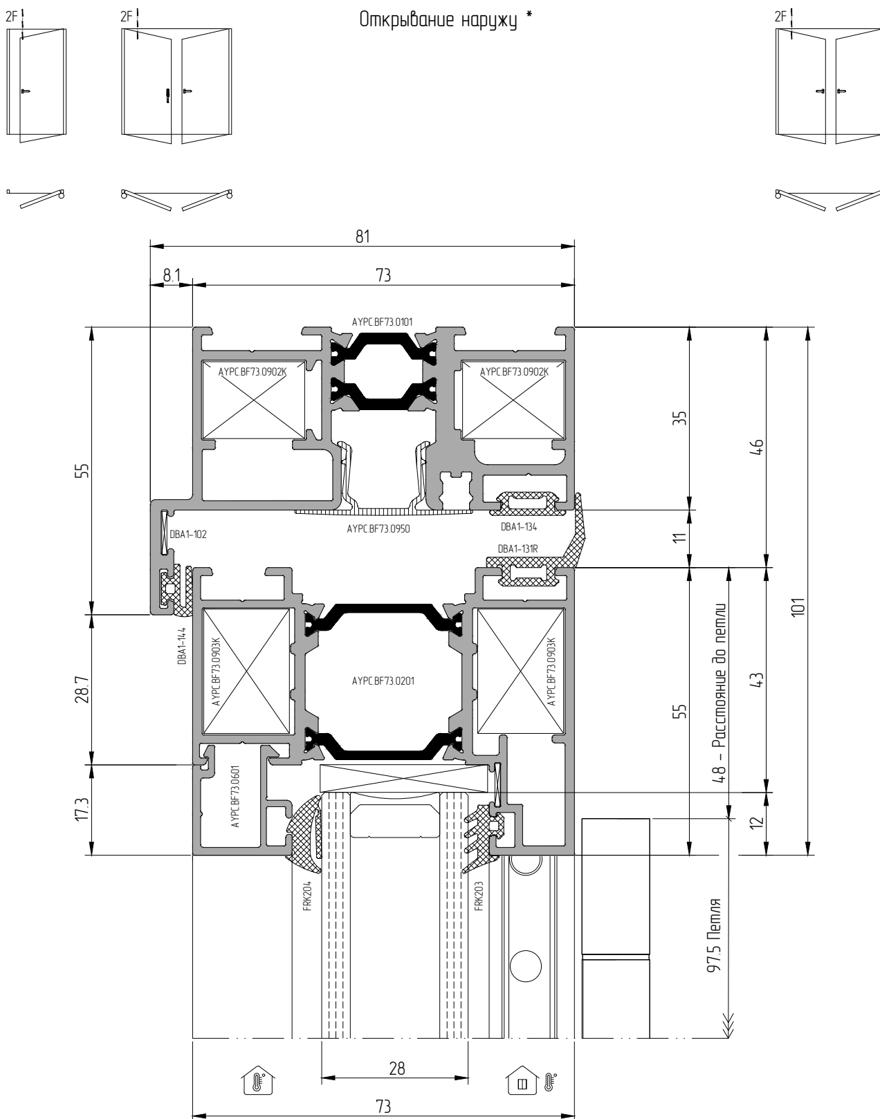
Сечение 2 – Верхний узел F.1 — Одностворчатые и двустворчатые двери. Верхний узел. Узкая створка АУРС.BF73.0201
