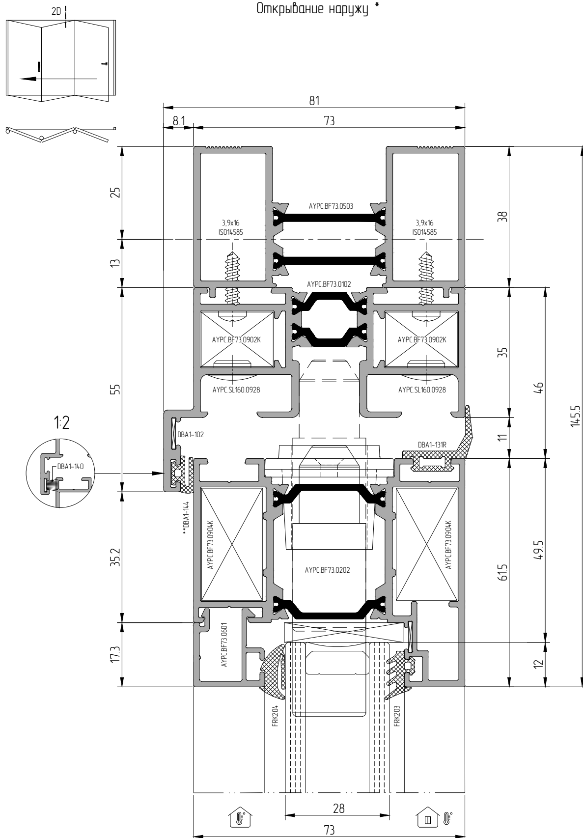
Сечение 2 – Верхний узел D.2 – Рама АУРС.BF73.0102 со шпингалетом и вент. профилем. Стандартная створка АУРС.BF73.0202
