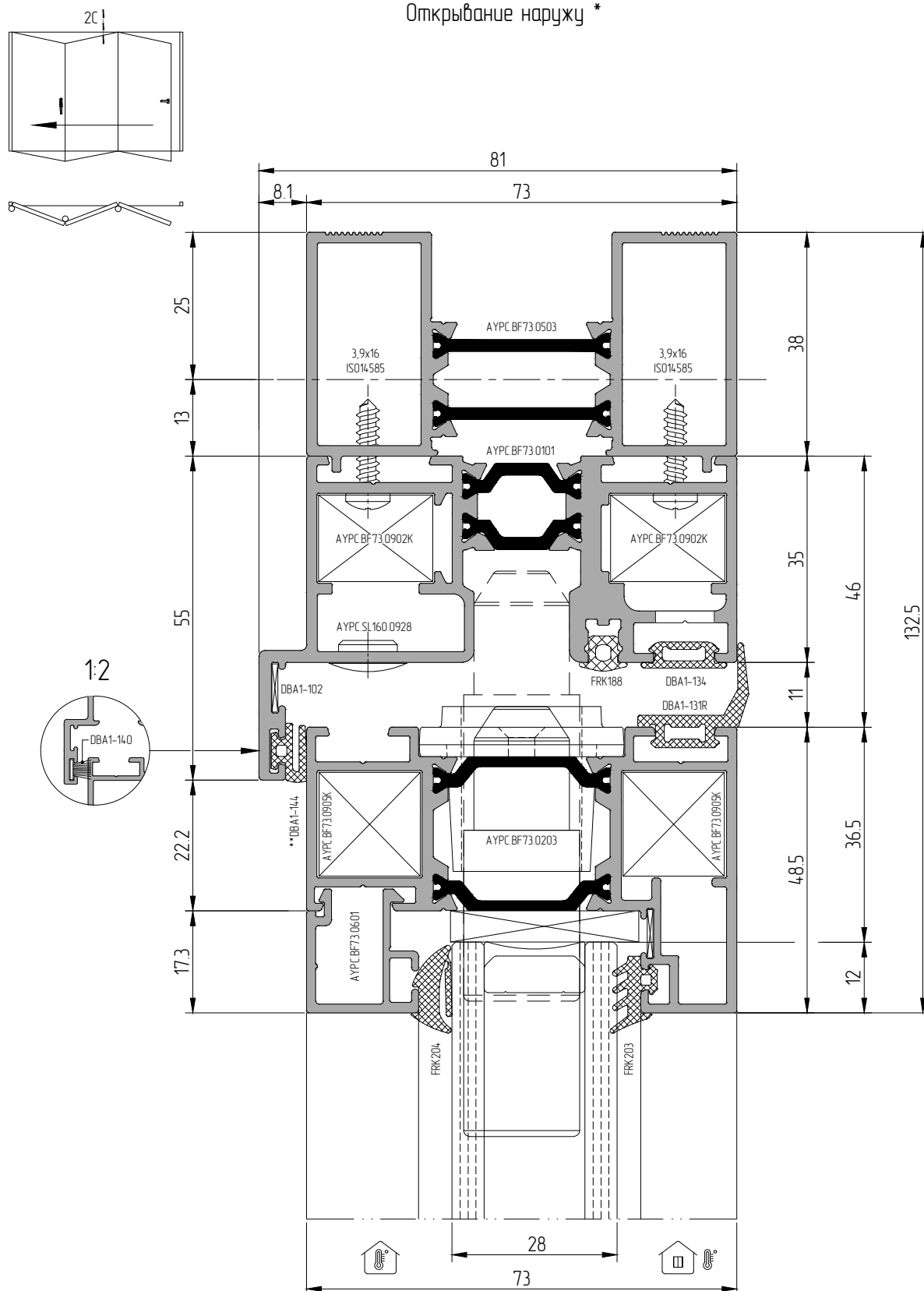
Сечение 2 – Верхний узел С.3 — Рама АУРС.BF73.0101 со шпингалетом и вент. профилем. Сверхузкая створка АУРС.BF73.0203
