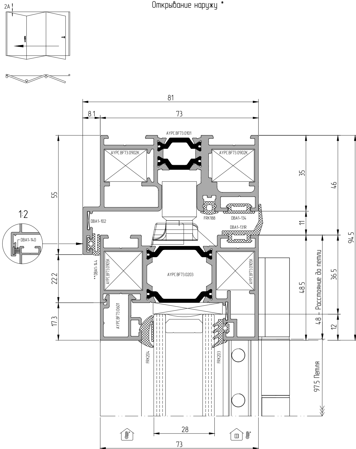
Сечение 2 – Верхний узел А.3 — Рама АУРС.BF73.0101 с направляющим роликом. Сверхузкая створка АУРС.BF73.0203
