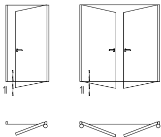
Сечение 1 – Нижний узел I.1 — Одностворчатые и двустворчатые французские двери. Нижний узел. Узкая створка АУРС.BF73.0201 Открывание наружу *
