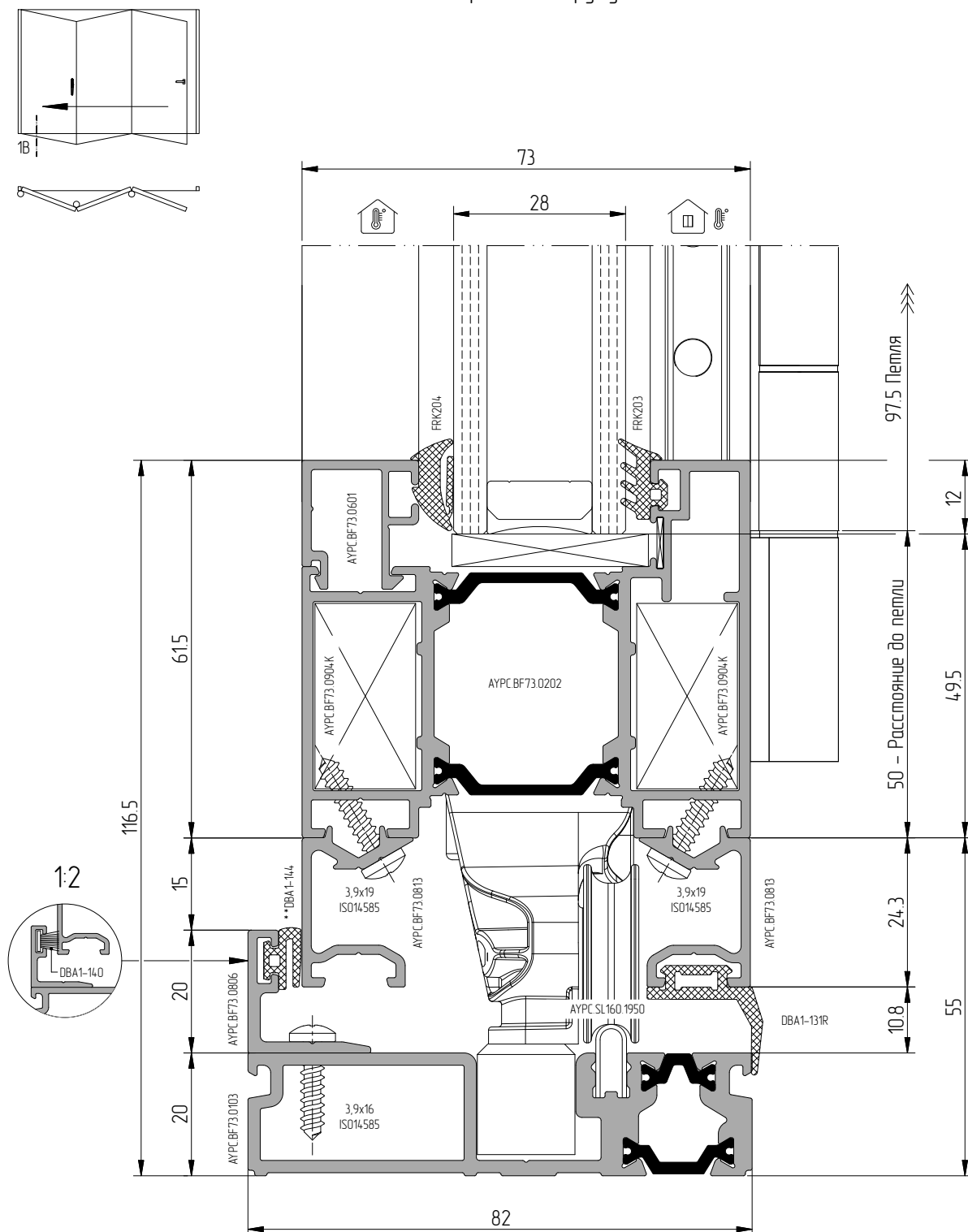
Сечение 1 – Нижний узел В.2 — Низкий порог АУРС.ВФ73.0103 с опорным роликом. Стандартная створка АУРС.ВФ73.0202
