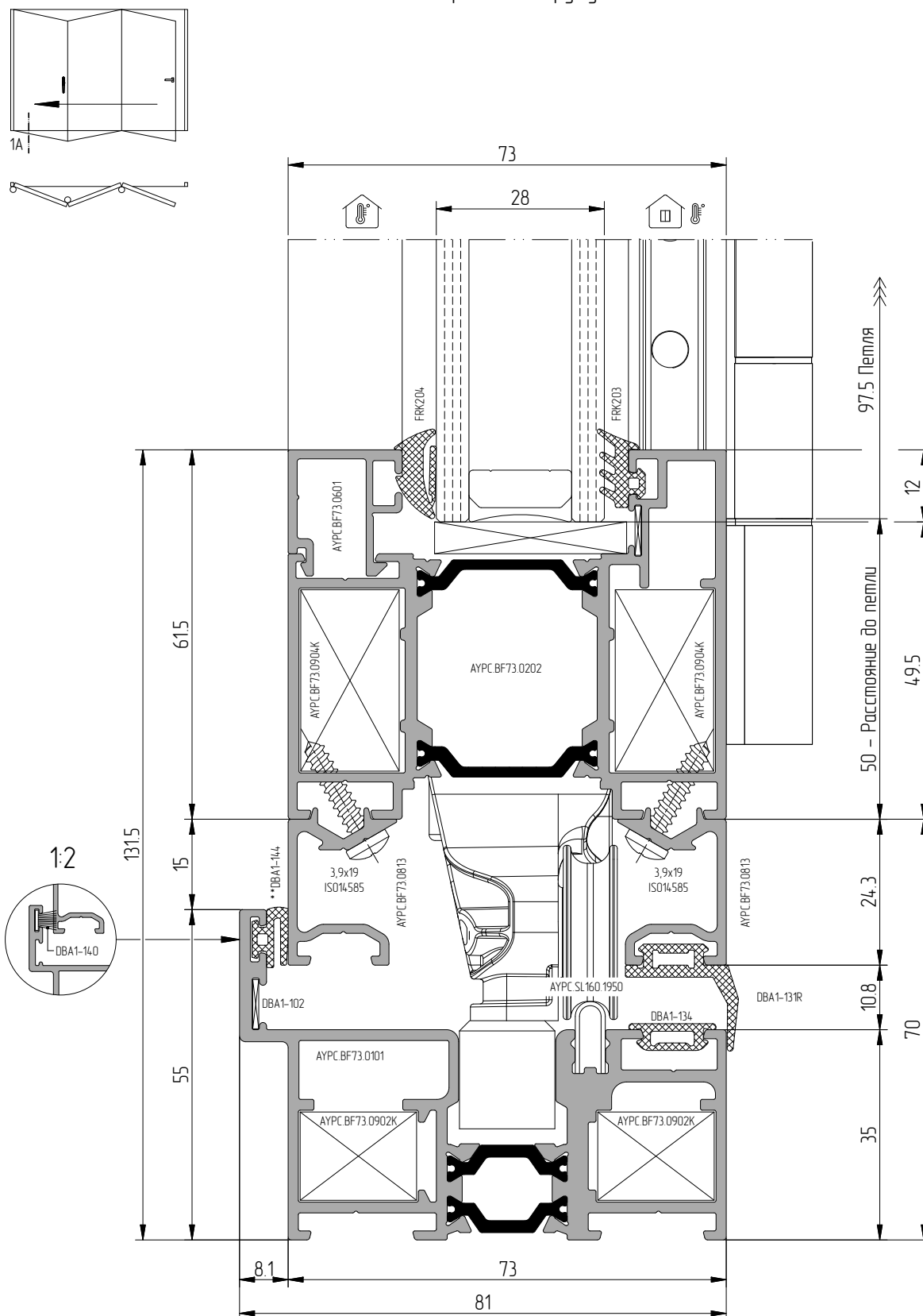
Сечение 1 – Нижний узел А.2 — Рама АУРС.BF73.0101 с опорным роликом. Стандартная створка АУРС.BF73.0202
