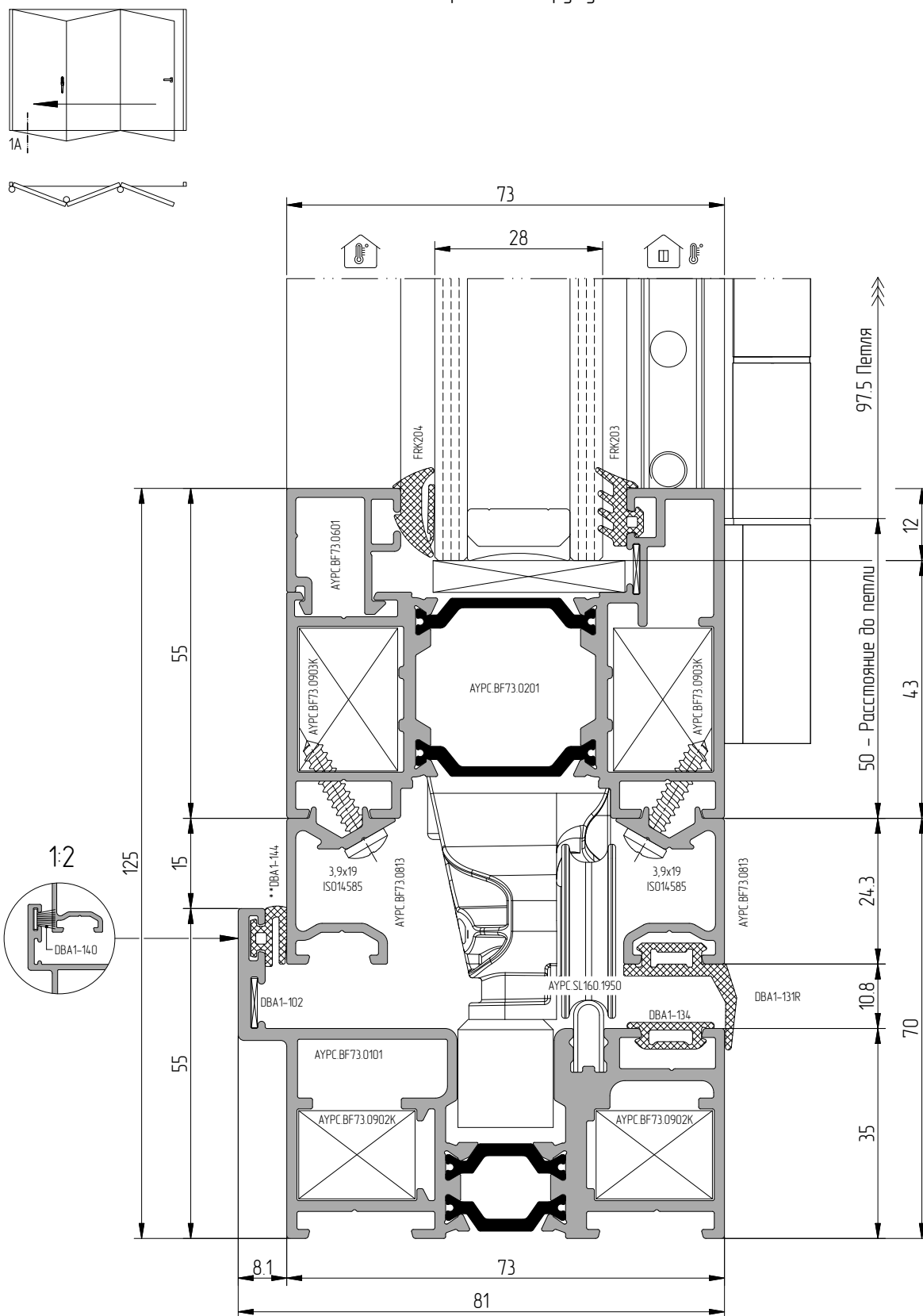
Сечение 1 – Нижний узел А.1 — Рама АУРС.BF73.0101 с опорным роликом. Узкая створка АУРС.BF73.0201
