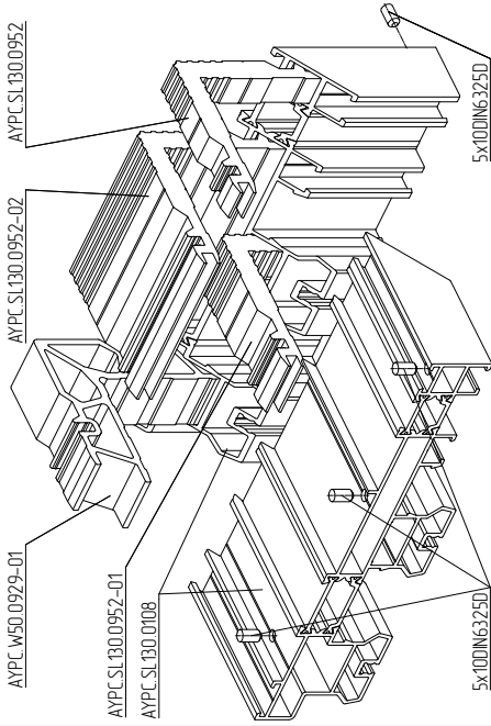
Угловое соединение профилей рамы АУРС SL130.0108
