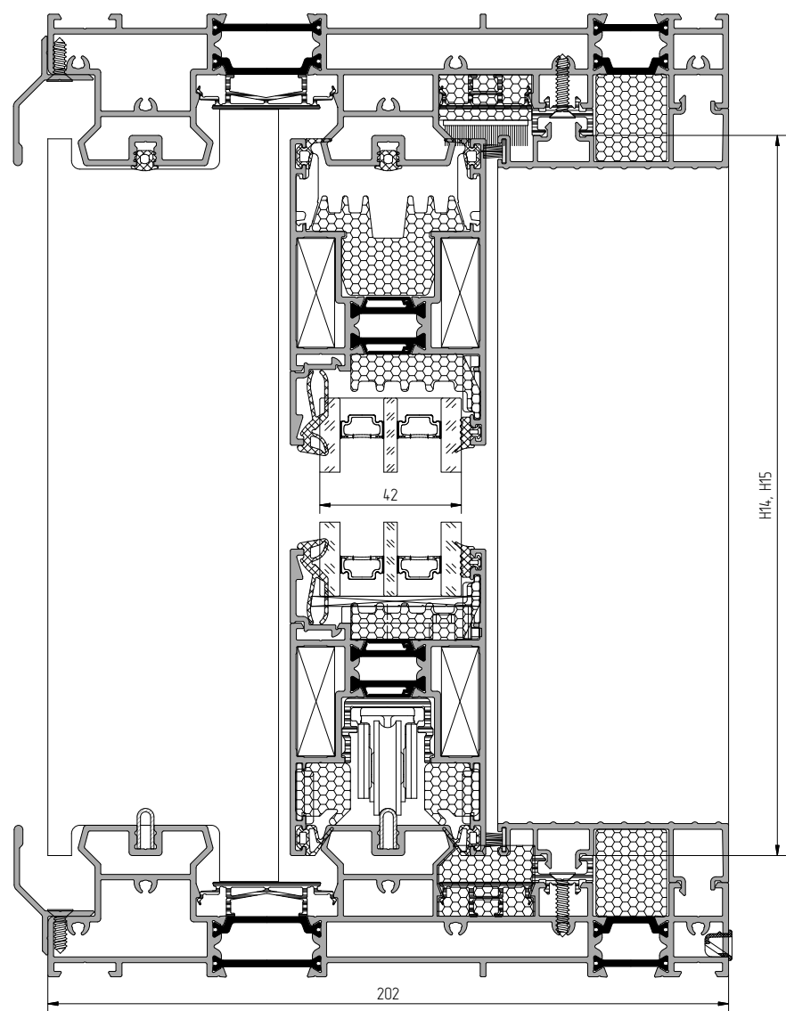
Вертикальные сечения
