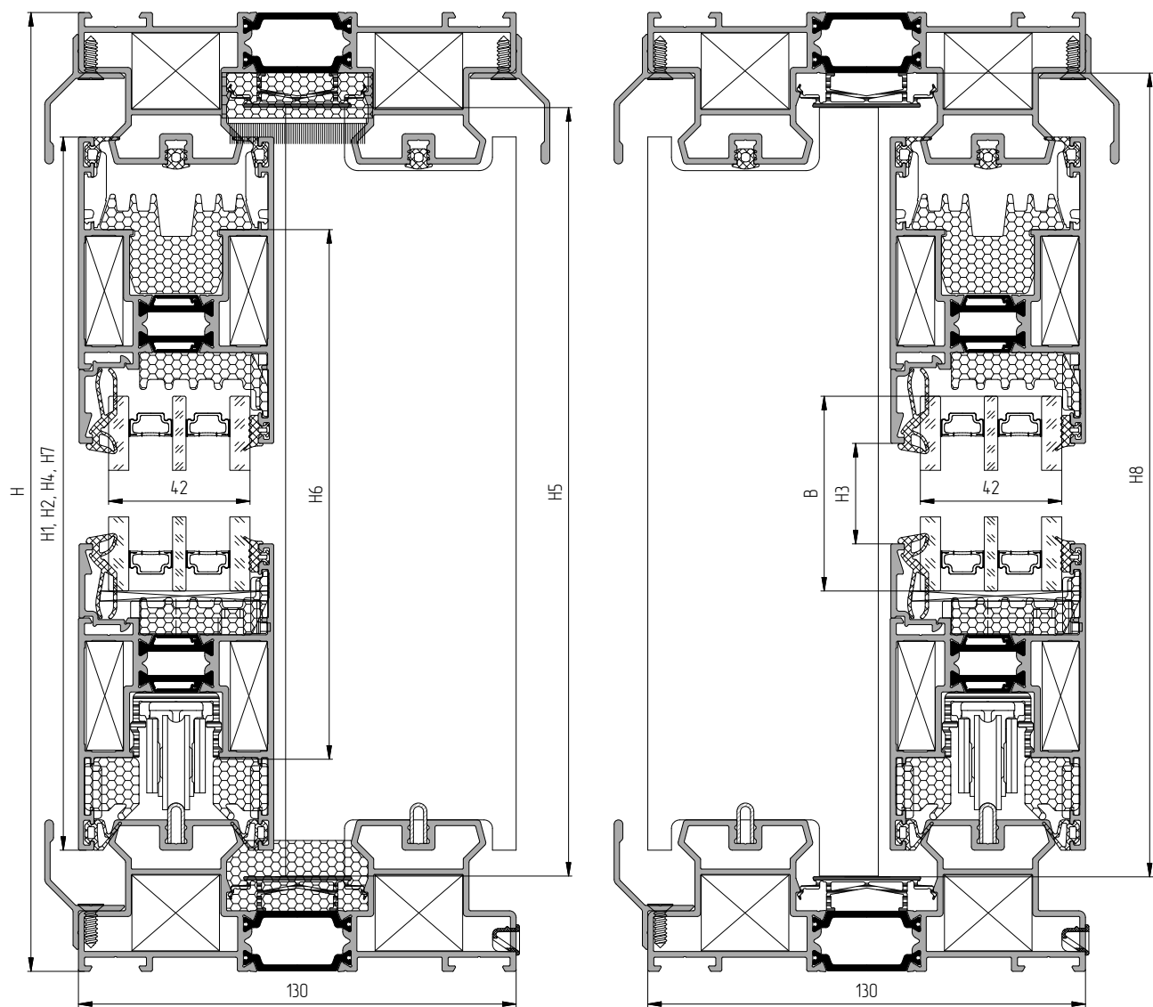
Вертикальные сечения
