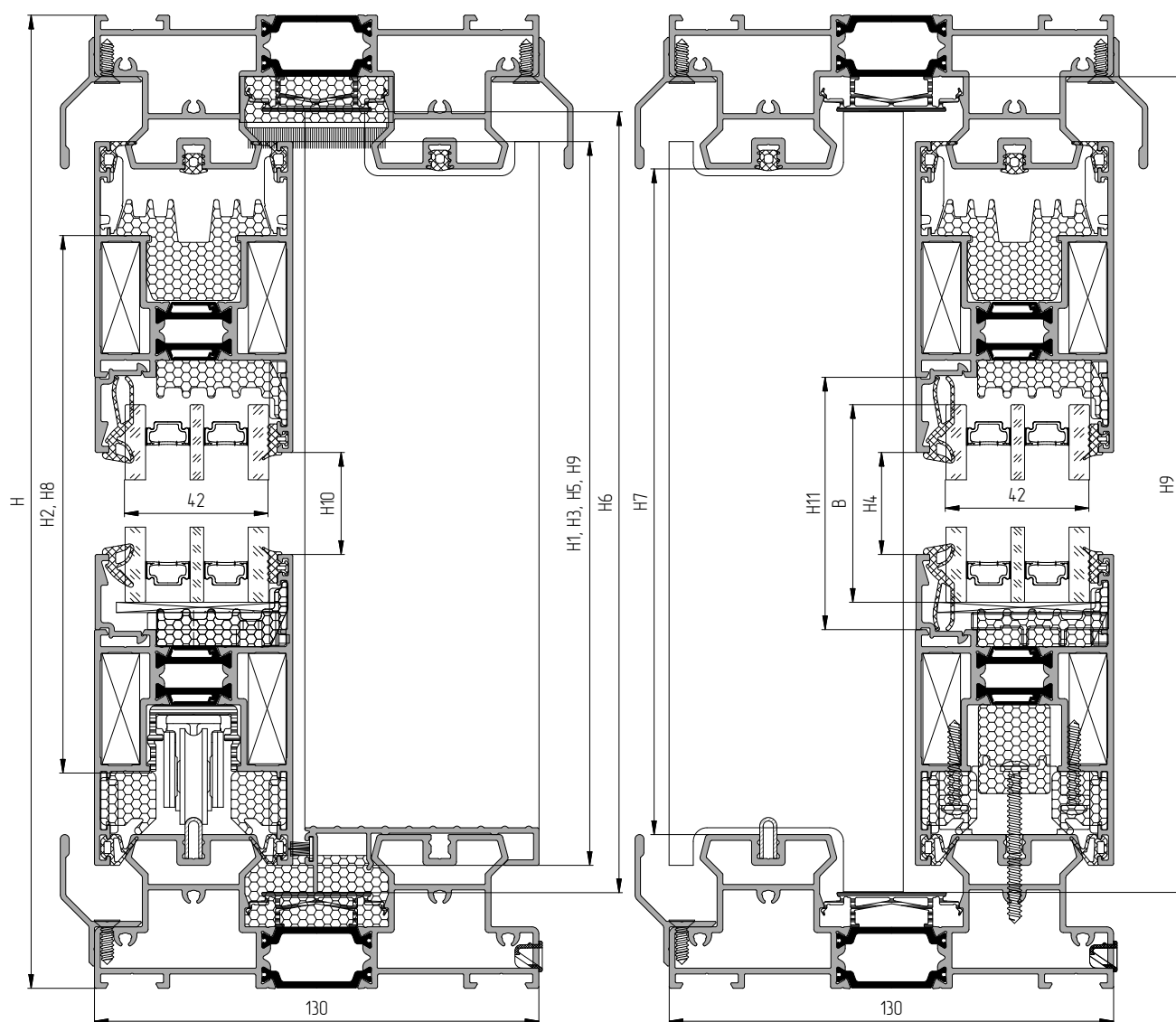
Вертикальные сечения
