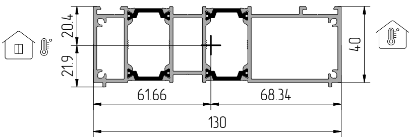
Профиль доборный АУРС.SL130.0509
