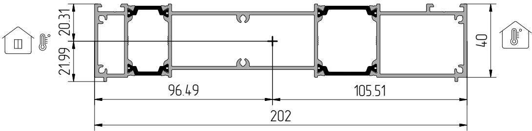
Профиль усилителя АУРС.SL130.0702
