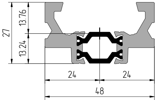
Профиль усилителя АУРС.SL130.0702
