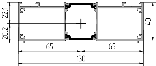
Профиль доборный АУРС.SL130.0508
