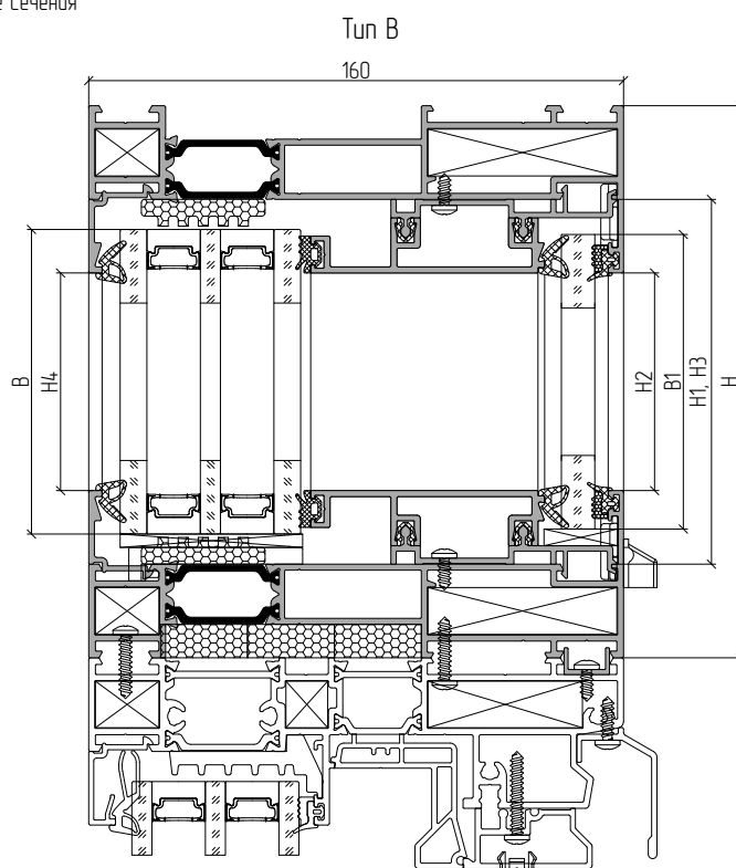
Горизонтальные сечения
