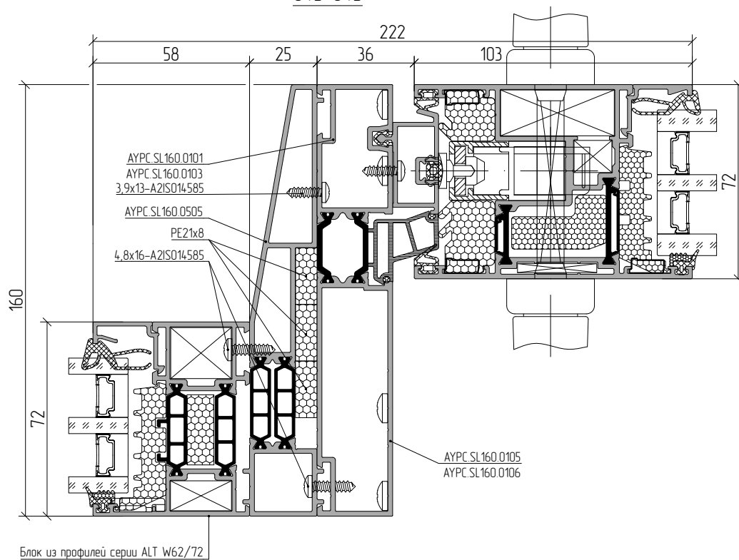
84b-84b
