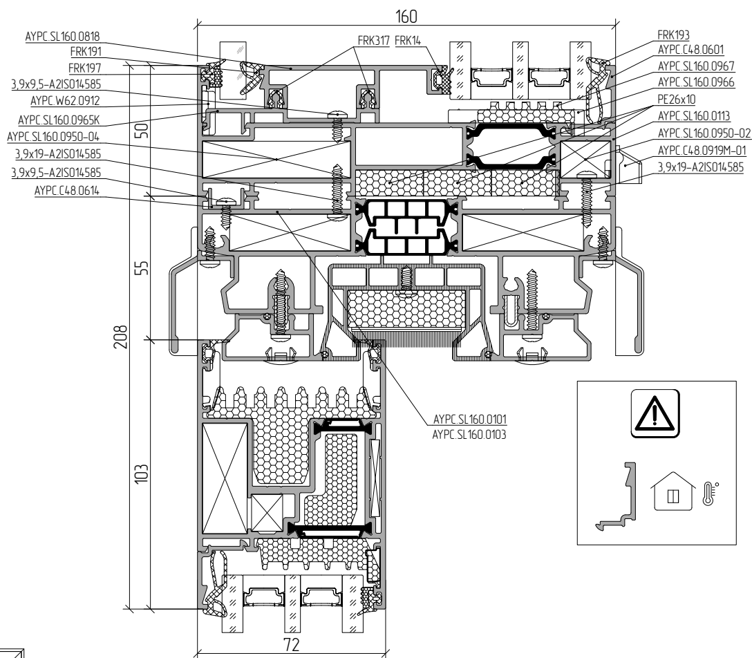
85b-85b
