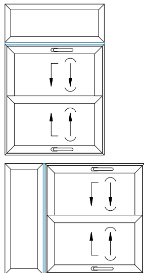
Схема обработки профиля адаптера АУРС.SL130.0502 и профилей рамы АУРС.SL130.0101, АУРС.SL130.0102, АУРС.SL130.0106
